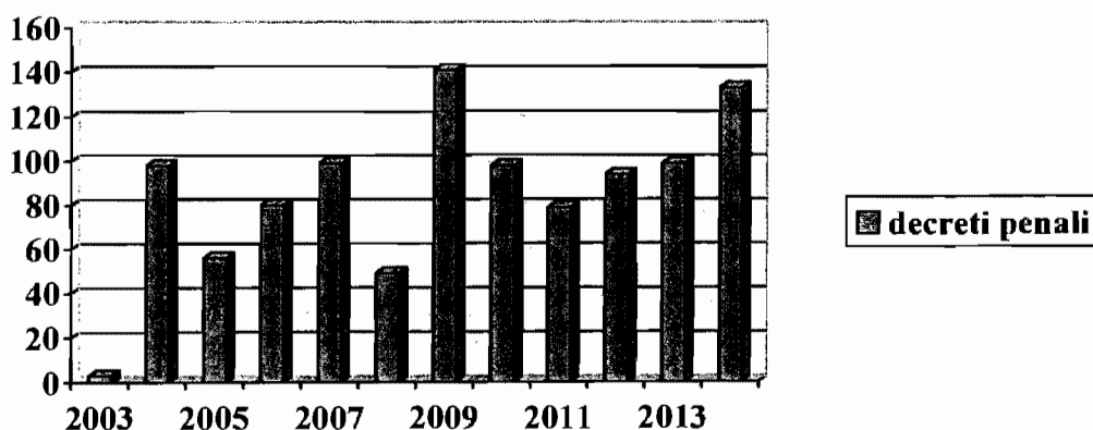
ISTOGRAMMA
