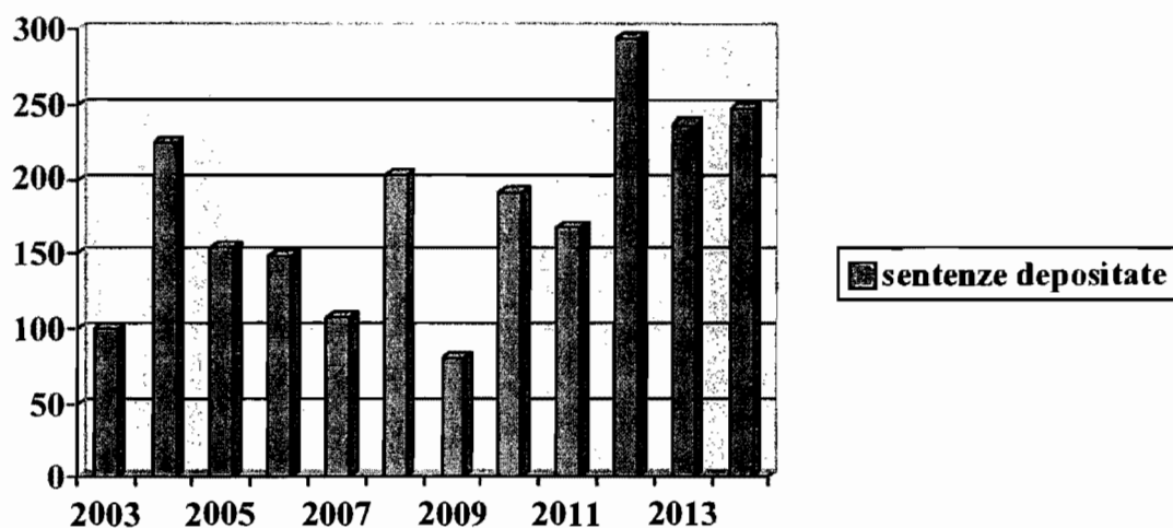
ISTOGRAMMA
