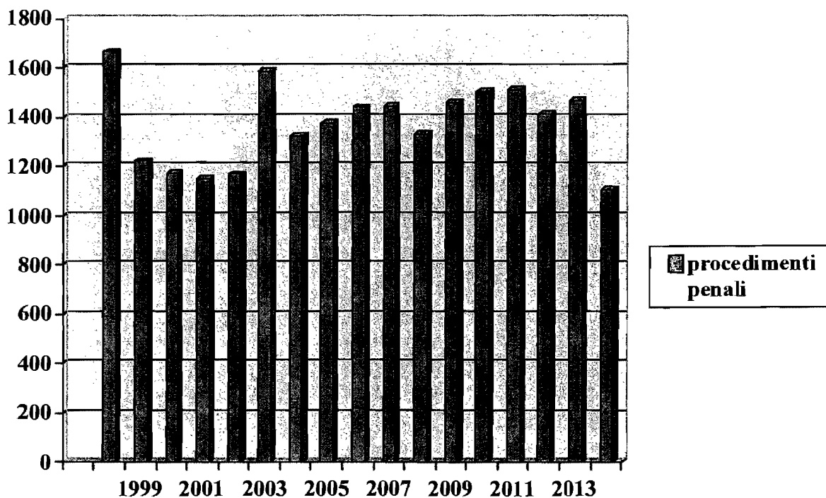
GRAFICO N. 1 - ISTOGRAMMA
