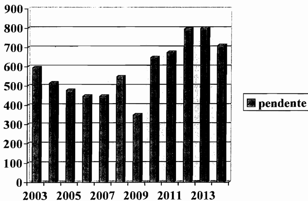
ISTOGRAMMA
